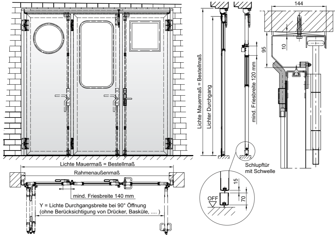
Montage ohne Sturz (gez. außen öffnend) in und vor der Laibung möglich
