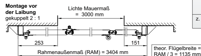
Verglasungsaufteilungen, weitere Aufteilungen möglich
