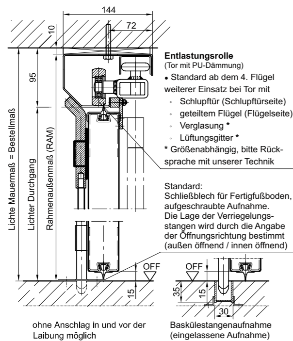
Montage ohne Sturz (gez. außen öffnend) in und vor der Laibung möglich
