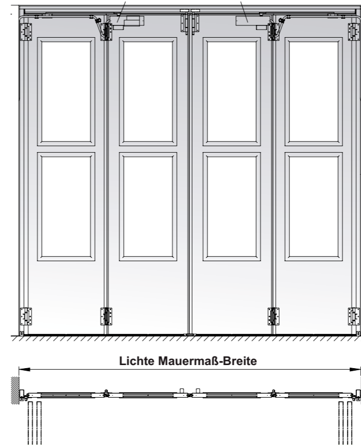
Antrieb „Ditec Dor 1BHS“
