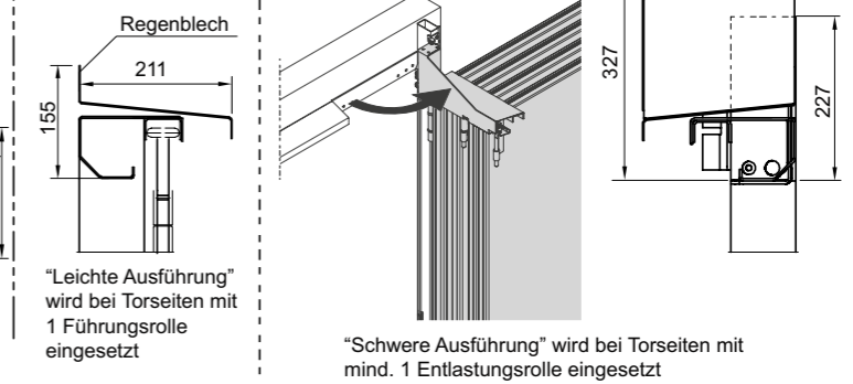
Montage vor der Laibung 180° Öffnung
