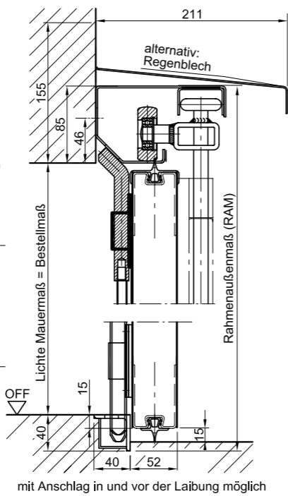
Montage vor der Laibung (gez. 90° nach außen öffnend)
