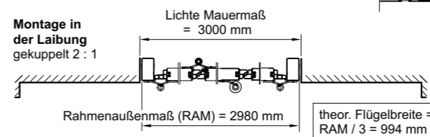
Montage vor der Laibung gekuppelt 2 : 1
