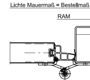
Montage In der Laibung
