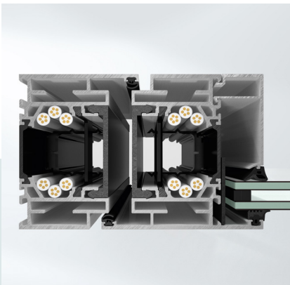
Thermisch getrennter Brandschutz: Neue falzoffene Profilgeometrie
