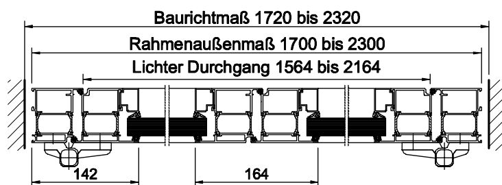
mit Verglasung und Sprosse (nach außen öffnend) Darstellung Gangflügel DIN links; DIN rechts spiegelbildlich
