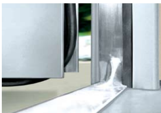
Hoogwaterdeur van Teckentrup. Door de slang op te pompen, wordt een waterdichte afsluiting bereikt.
