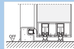
Anslagströskel och dubbel uppfäll- och nedsänkbar golvtätning (ej för flykt- och räddningsvägar)
