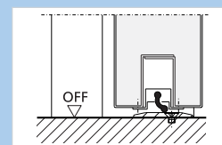
Släplista med tröskelplatta
