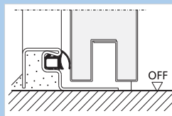
Anslagströskel (ej för flykt- och räddningsvägar)
