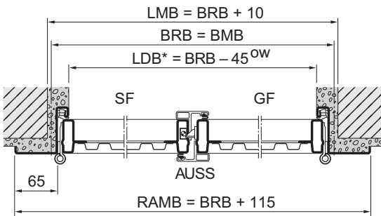
Außenanschlag – nach außen öffnend
