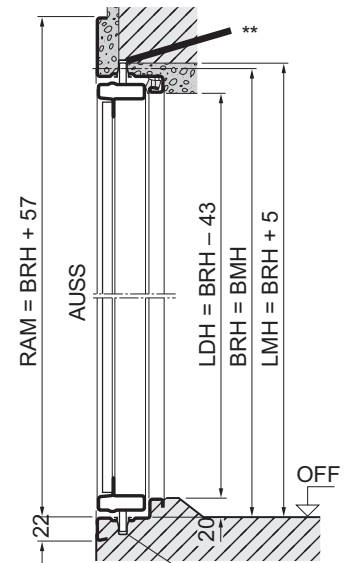
mit unterem Anschlag
