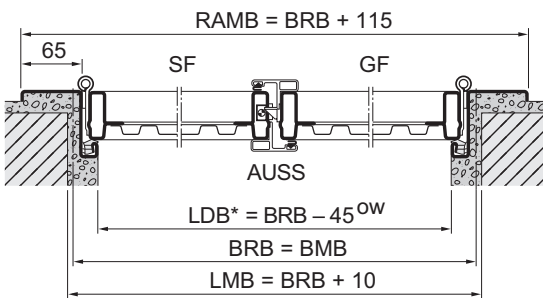
Außenanschlag – nach außen öffnend
