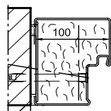
Blokkozijn Type 4.2
