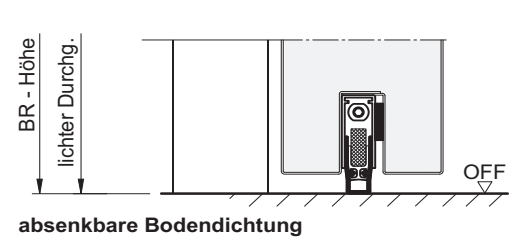
absenkbare Bodendichtung
