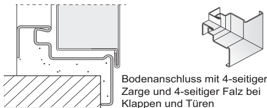
„Teckentrup“ - Doppel-Schleifdichtung Zarge mit Bodeneinstand zwingend erforderlich
